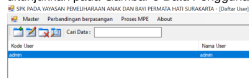
Gambar 6. Data Pengguna
